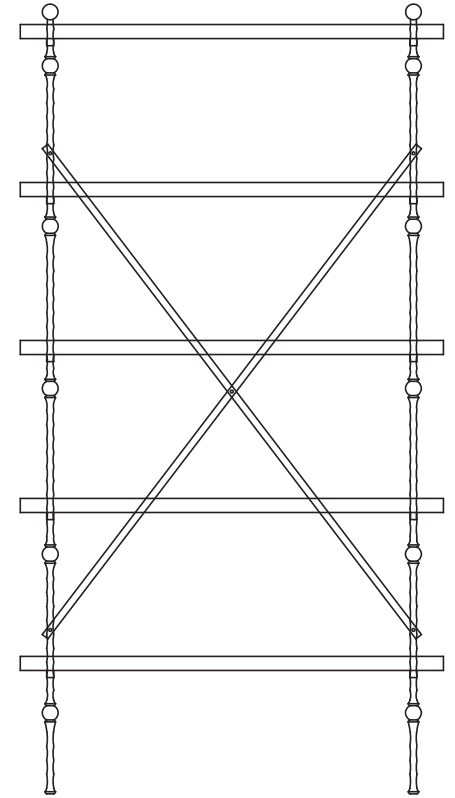
BOOKCASE H: 2240 W: 1200 D: 460
