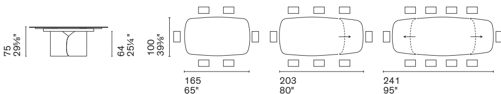
CS4153-S 165 / CS4153-S 165 MTO
