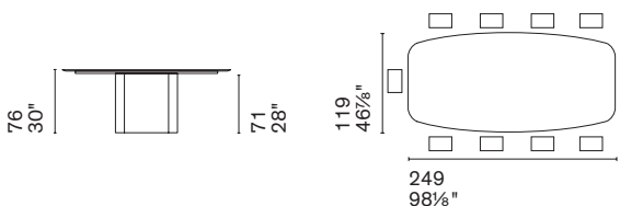
CS4153-FB 250 / CS4153-FB 250 MTO
