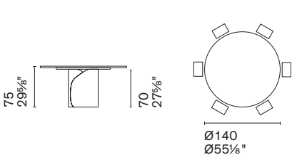
CS4153-FD 140 / CS4153-FD 140 MTO
